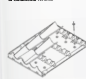
9.3 "Realizzazione dello strato di ventilazione e dello strato di isolamento termico"
